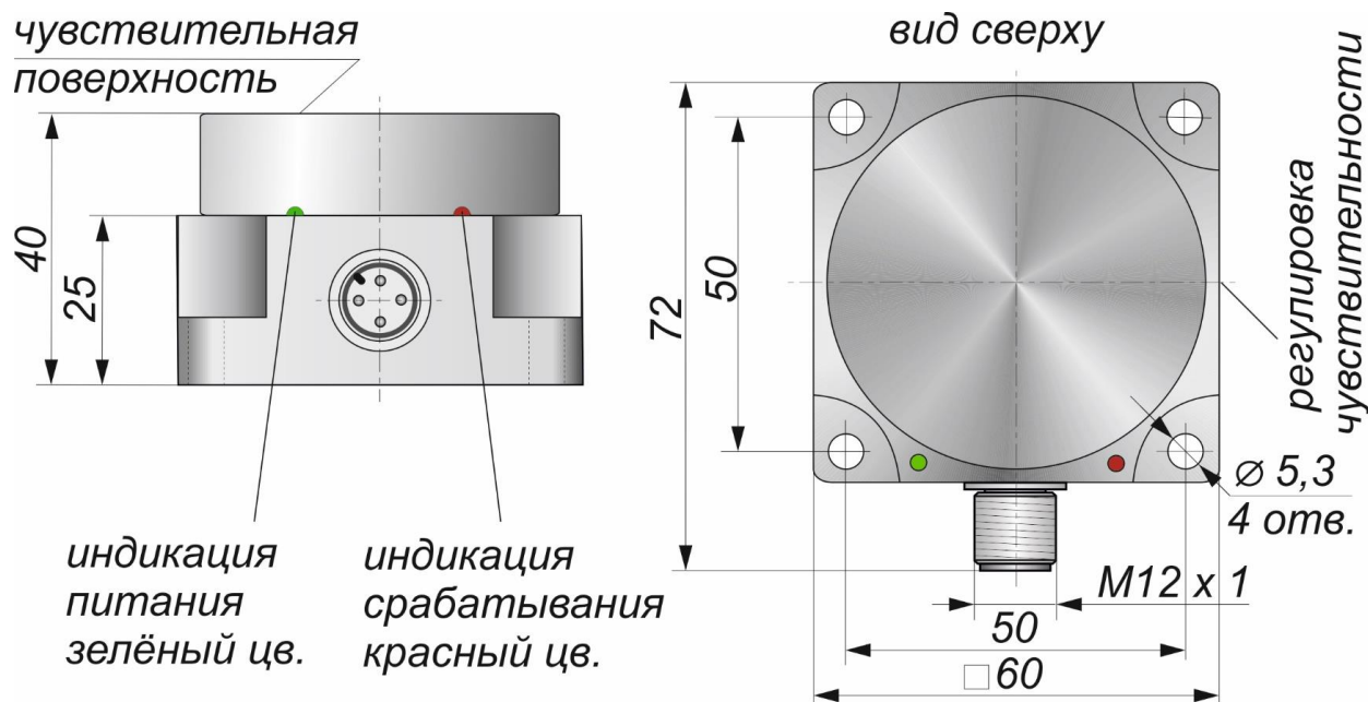
Габаритный чертеж
